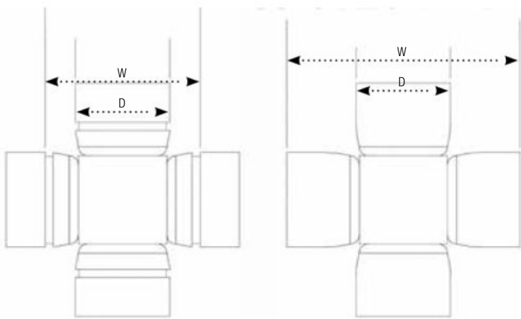
Type 1: Emplacement de clips à l'intérieur Type 1: Inside snap rings
