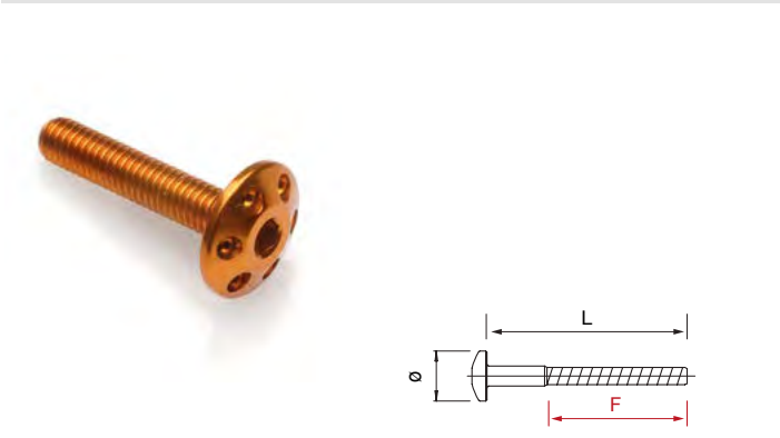
Drilled bolts - Tornillos agujereados
